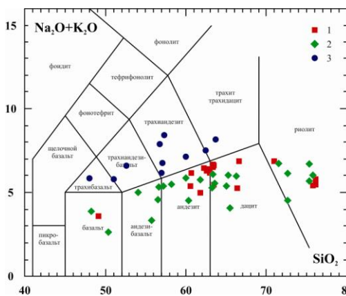
Рисунок 8 - Соотношение содержаний \text{SiO}_2 - ( \text{Na}_2\text{O} + \text{K}_2\text{O} ) в раннекембрийских вулканитах олдындинской свиты на классификационной диаграмме [Le Maitre et al., 1989] 1 – вулканиды Еравнинской ВТС, 2 – вулканиды Олдындинской ВТС, 3 – вулканиды Кыджимитской ВТС
