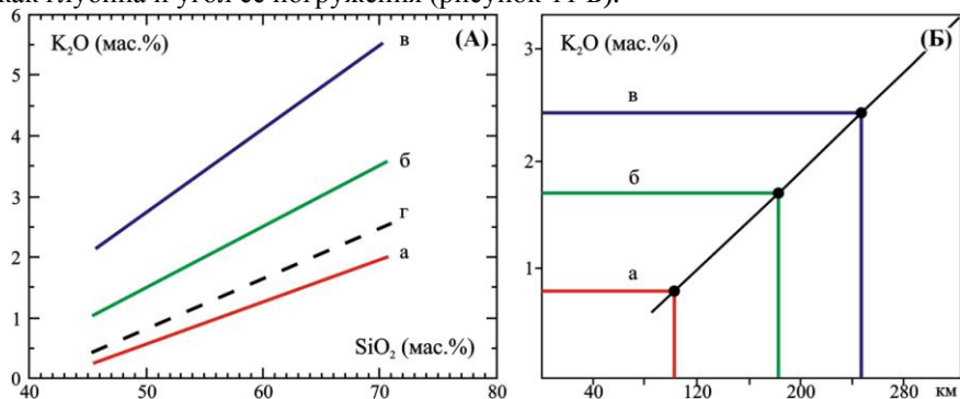
Рисунок 11 – А) Вариационная диаграмма содержаний \text{K}_2\text{O} относительно \text{SiO}_2 в раннекембрийских вулканитах Еравнинской (а), Олдындинской (б), Кыджимитской (в) ВТС и лавах вулканов Курильской островной дуги (г), по [Чашин, Мартынов, 2011]. Б) График корреляции \text{K}_2\text{O} (при \text{SiO}_2=55\% ) в раннекембрийских вулканитах Еравнинской (а), Олдындинской (б), Кыджимитской (в) ВТС с глубиной залегания зоны субдукции, по [Dickinson, Natherton, 1967]
